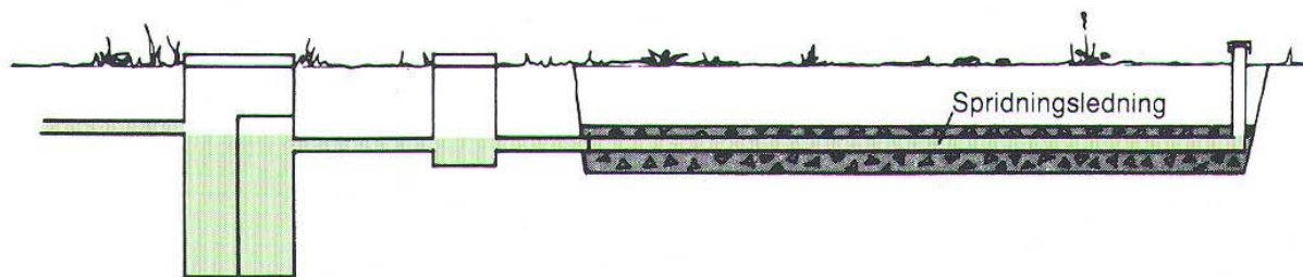
Slamavskiljare Fördelningsbrunn
