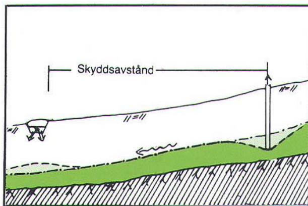
Normalfallet. Anläggningen placerad nedströms vattentäkten.
